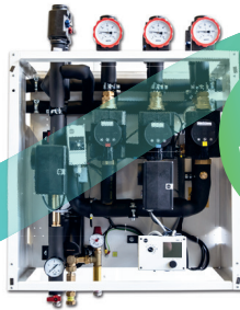
Fernwärme-Übergabestation Taurus-Serie
